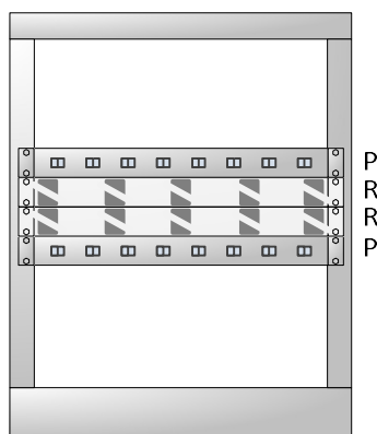
Abbildung 4: Aufbau LWL Patchpanel/Rangierpanel PRRP
