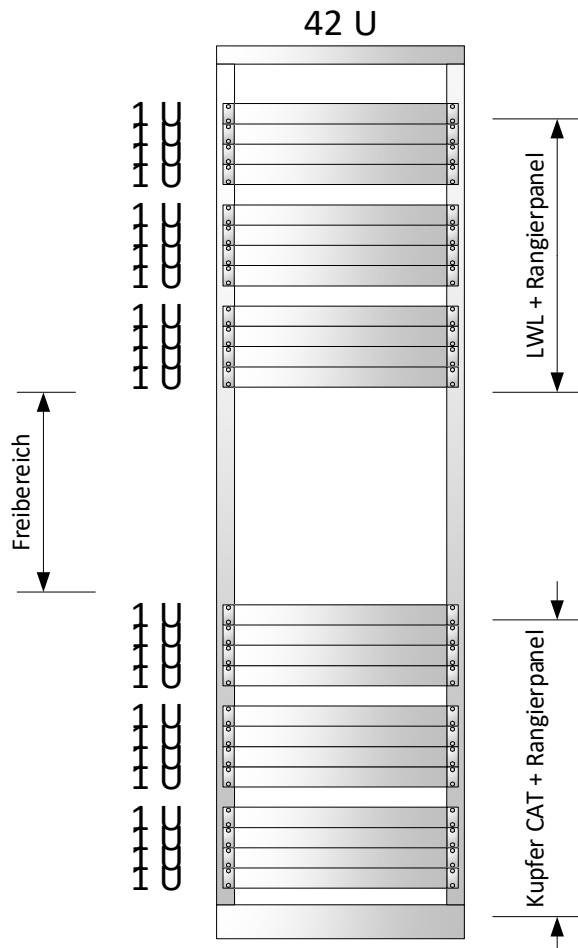
Abbildung 7:Abbildung Mischverkabelung
