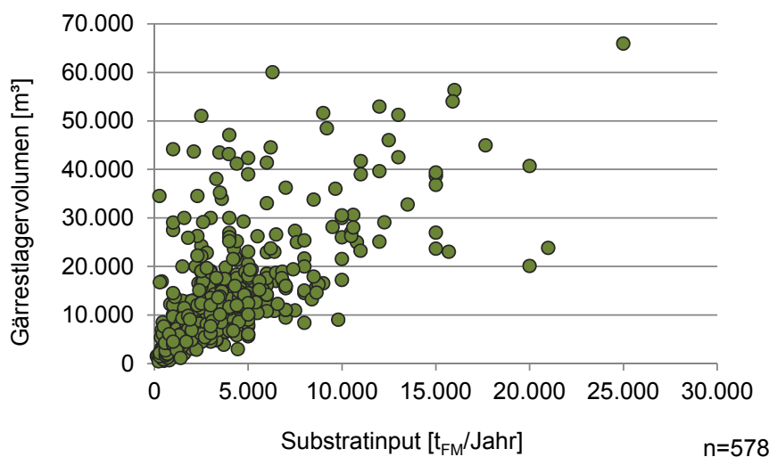
Abb. 3-25: Gärrestlagervolumen in Abhängigkeit vom Substratinput (Betreiberbefragung DBFZ 2011/12)
