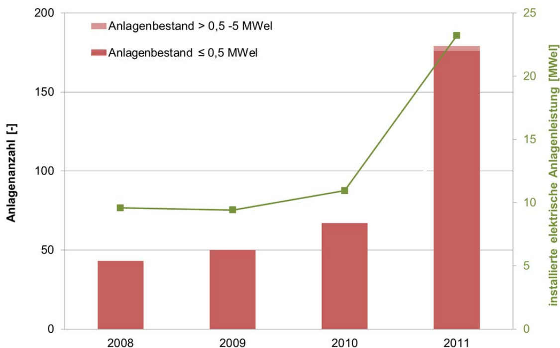
Abb. 2-17: Entwicklung des Anlagenbestandes und der installierten elektrischen Leistung nach Größenklassen von thermochemischen Vergasungsanlagen 5
